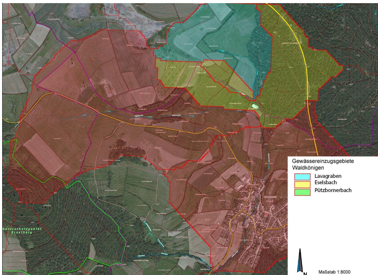
Abb. 2: Einzugsgebiete der für die Ortslage relevanten Gewässer 3. Ordnung
